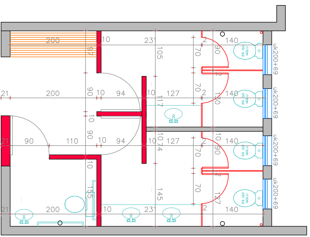
תכנית מוצעת
