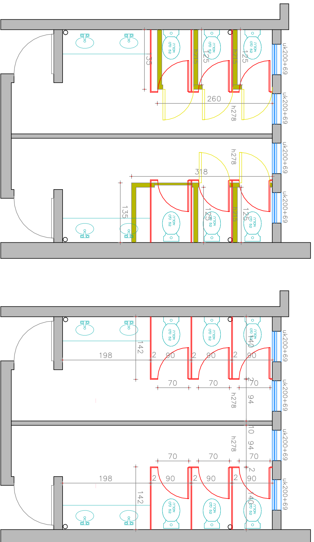
תכנית הריוסה
