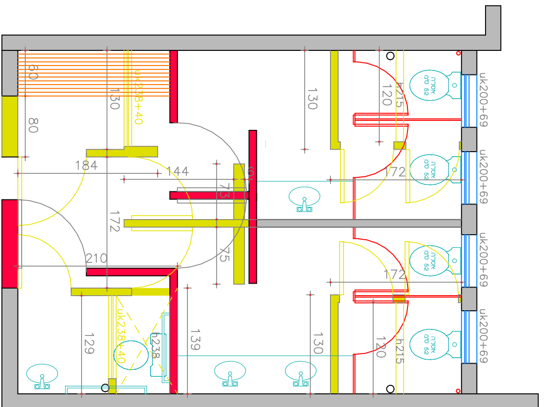
תכנית הריסה
