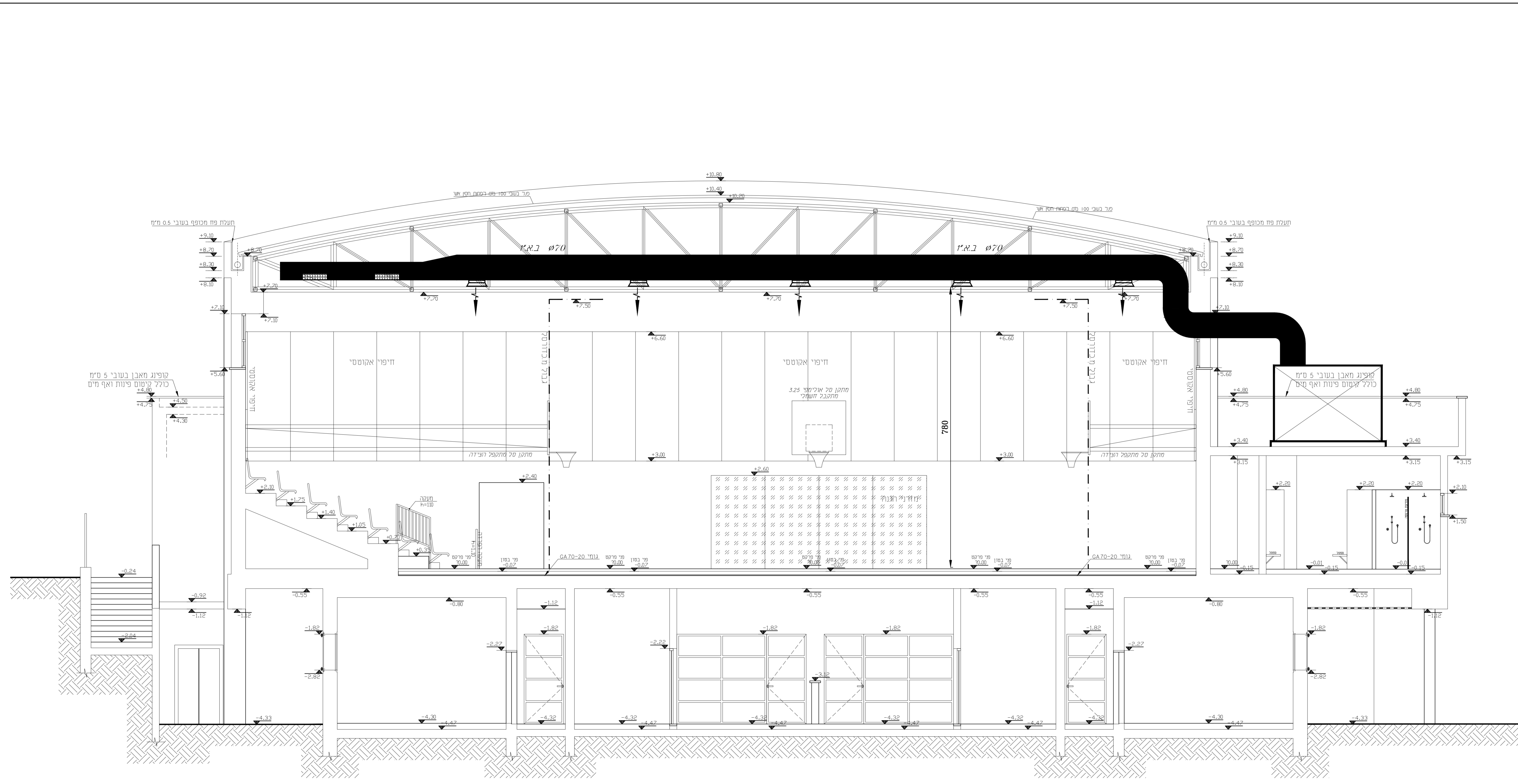
חתך א-א קני"מ 1:50
